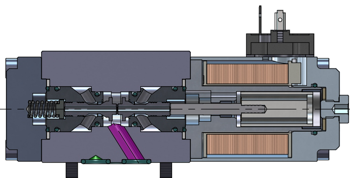
6通径剖面图
