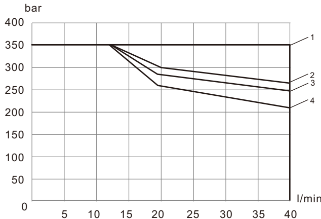
工作极限
