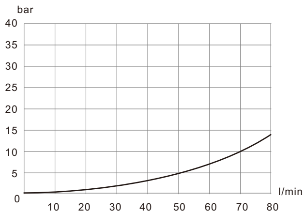
流量 - 压降
