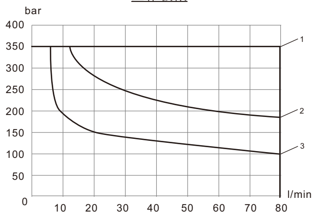
工作极限
