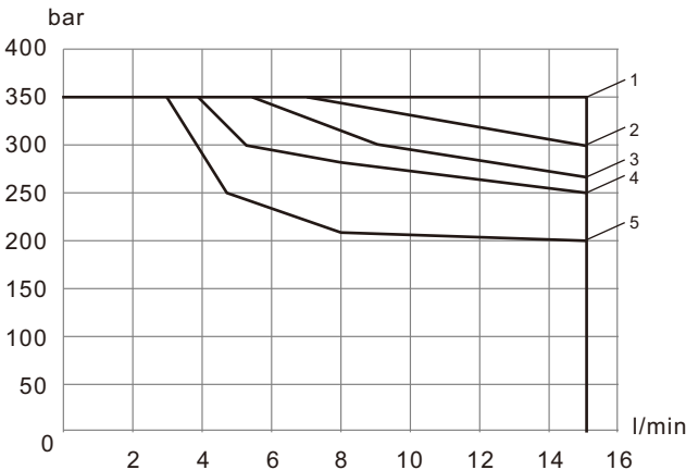
工作极限
